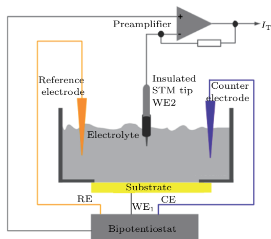
图 9 EC-STM 工作原理示意图, 双恒电位控制针尖和样品的电位
